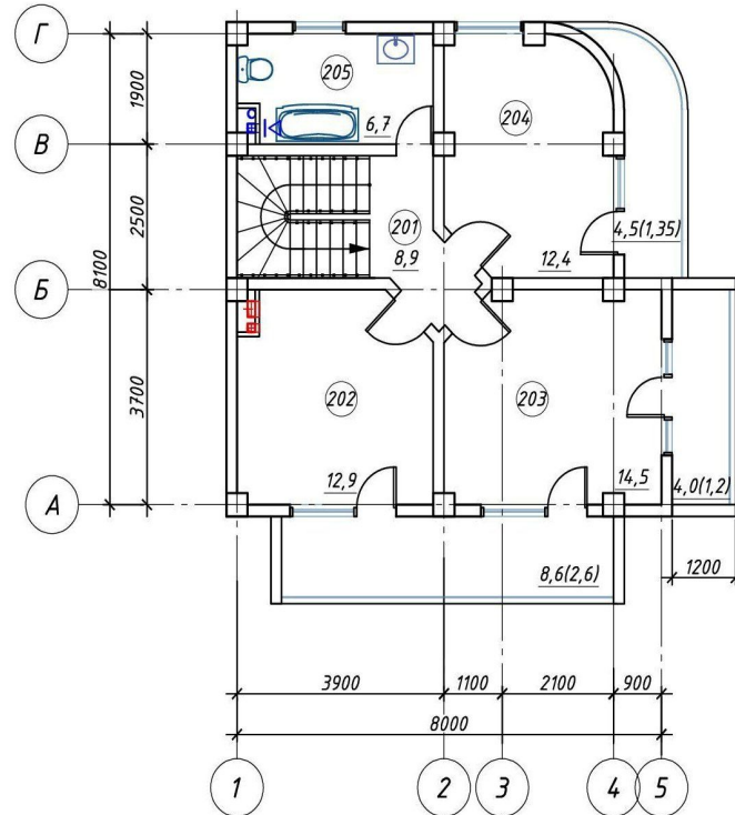
План второго этажа
