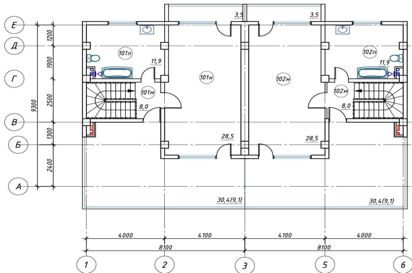
План третьего этажа
