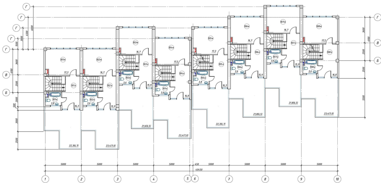
План третьего этажа
